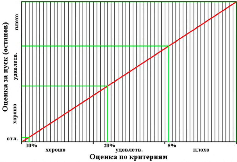
Рисунок А.3 – График определения оценки за качество пуска (останова) в зависимости от оценок по дополнительным критериям.
