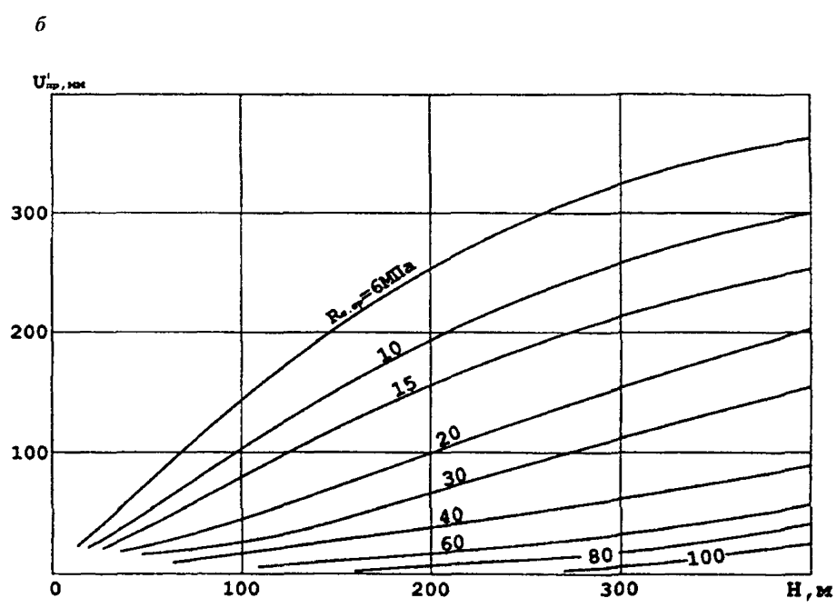
Рис. 8. Графики ( a – общий, б – для небольших глубин) смещений пород в присечных выработках вне зоны влияния собственного очистного забоя
