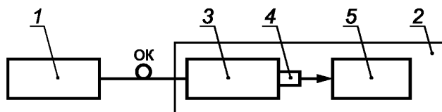
1 — проверяемый ОР; 2 — спектральная установка РЭСМ-ВС (СУ); 3 — монохроматор; 4 — фотоприемное устройство; 5 — регистратор, ОК — оптический кабель
