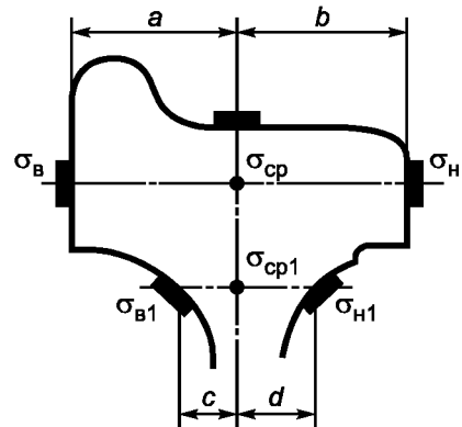
Рисунок А.6 — Схема приведения к плоскости круга катания ( \sigma_{cp} и \sigma_{cp1} ) напряжений замеренных ( \sigma_B , \sigma_H , \sigma_{B1} , \sigma_{H1} ) на боковых поверхностях обода (бандажа) и приободной части диска
