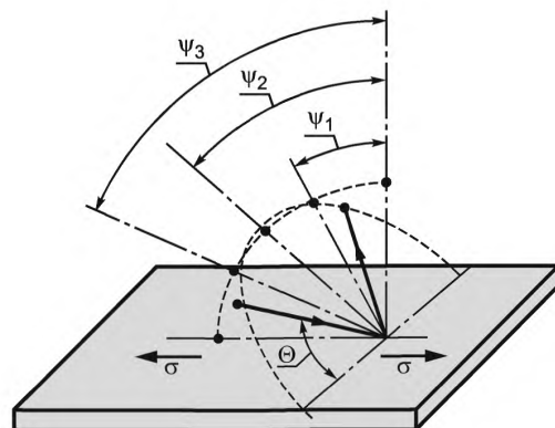
Рисунок 1 — Схема измерения для различных углов \psi
