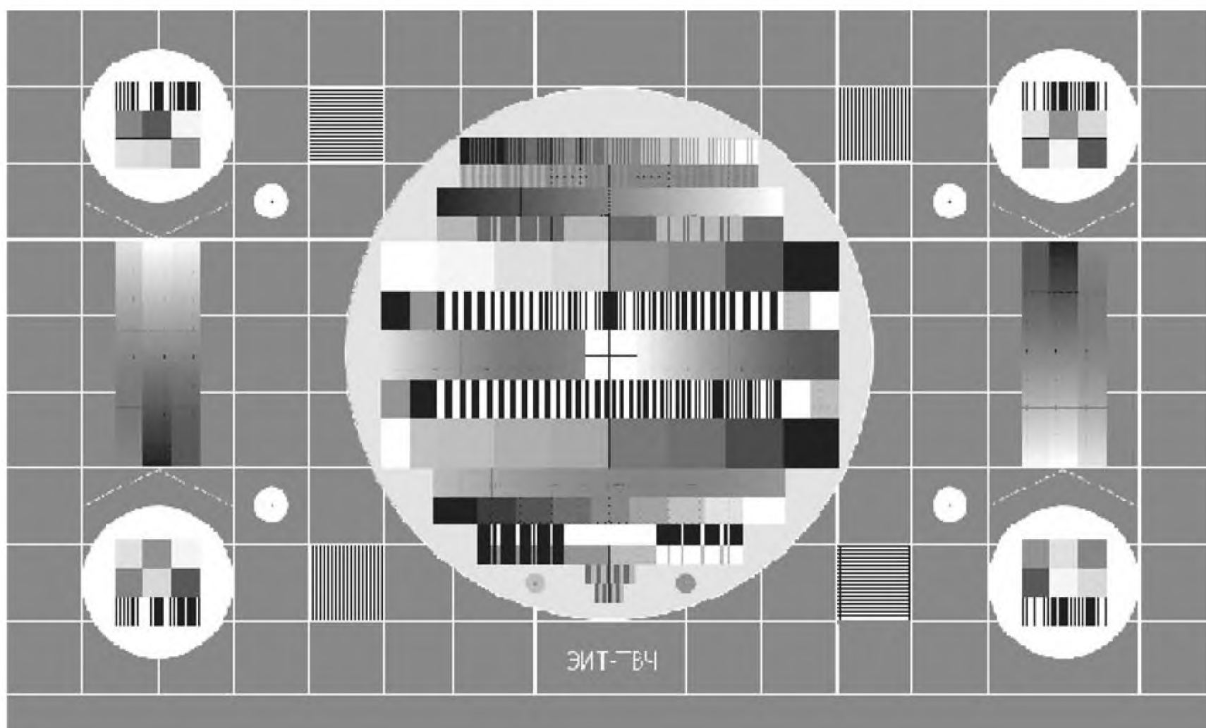
Рисунок А.3 — Электронная испытательная таблица для цифрового телевидения высокой четкости
