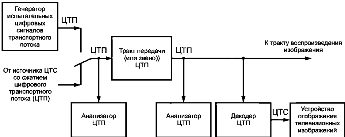
Рисунок 5 — Схема измерения параметров тракта передачи цифрового транспортного потока
