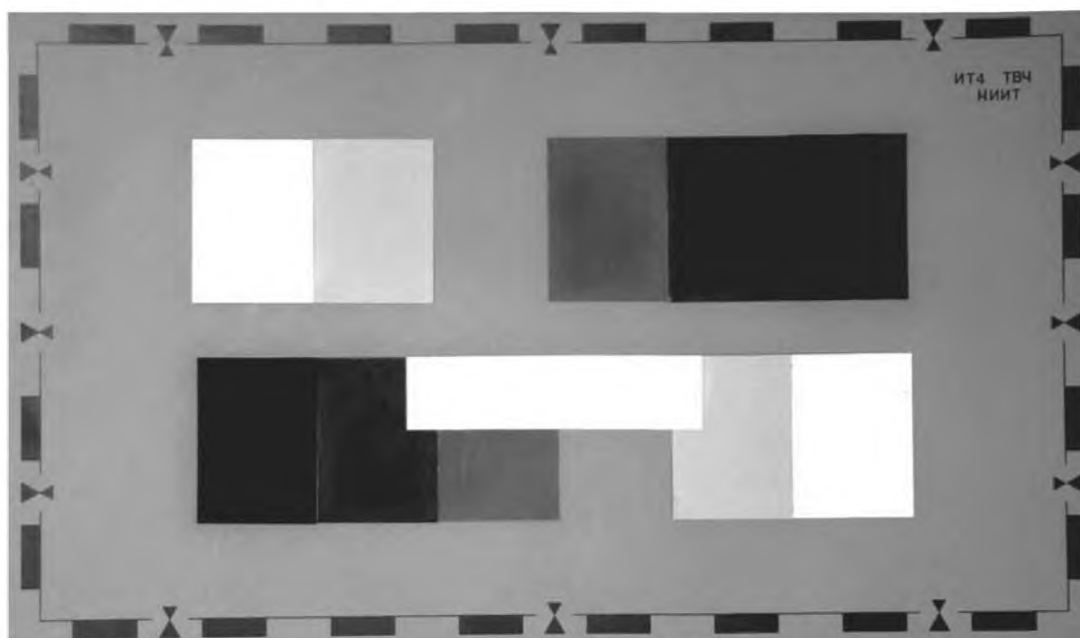
Рисунок А.2 — Таблица с градационными полями по яркости для оценки линейности световой характеристики телевизионных камер и тракта цифровой системы телевидения высокой четкости в целом
