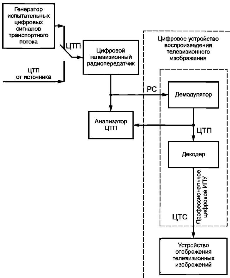
Рисунок 7 — Схема измерения параметров профессионального цифрового интегрированного приемного устройства
