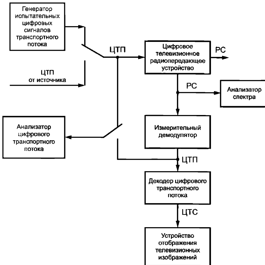
Рисунок 6 — Схема измерения параметров цифрового телевизионного радиопередающего устройства высокой четкости
