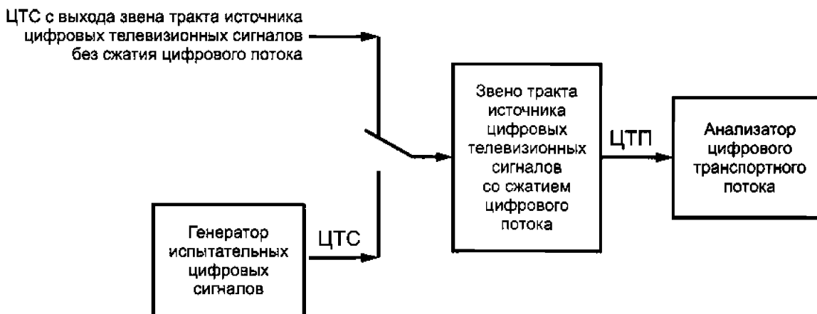
Рисунок 4 — Измерение параметров звена тракта источника цифровых телевизионных сигналов со сжатием цифрового потока
