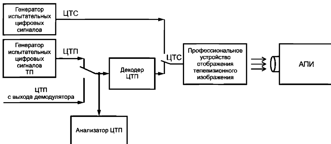
Рисунок 9 — Схема измерения характеристик и параметров тракта воспроизведения цифровых сигналов высокой четкости
