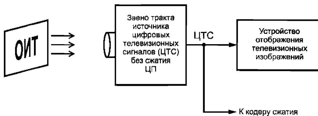
Рисунок 3 — Измерение параметров звена тракта источника цифровых телевизионных сигналов без сжатия цифрового потока
