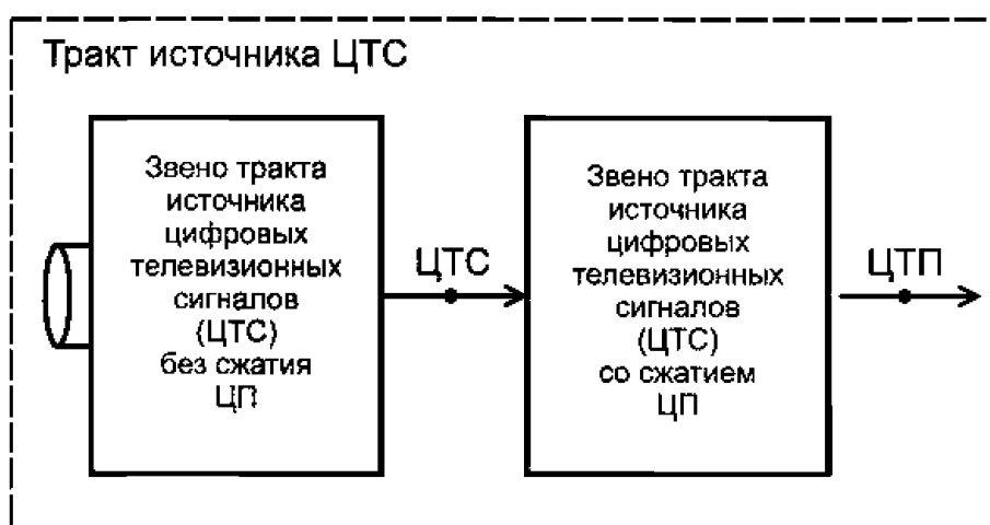
Рисунок 2 — Звенья тракта источника цифровых телевизионных сигналов
