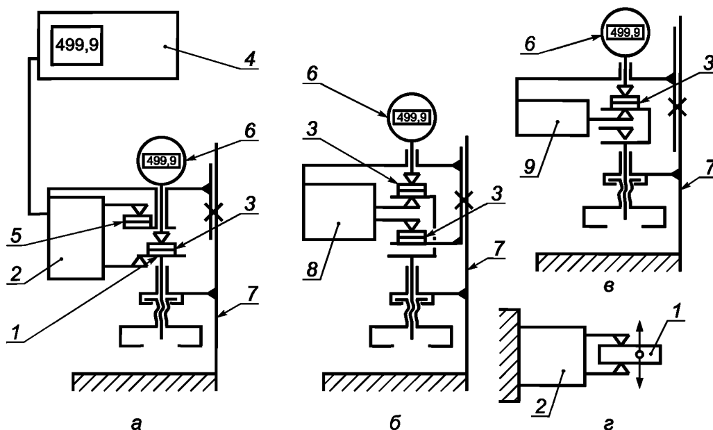
1 — стол; 2, 8, 9 — измерительное устройство; 3, 5 — концевая мера длины; 4 — цифровой электронный блок; 6 — цифровая измерительная головка; 7 — стойка
