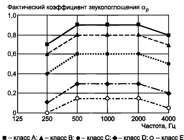
Рисунок 1 — Нормативные кривые, ограничивающие классы звукопоглощения
