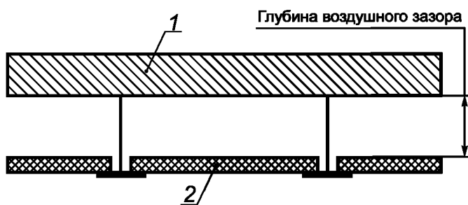
1 — поверхность помещения; 2 — звукопоглотитель
