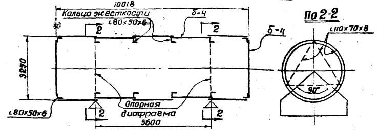
Резервуары 100 м 3 Н.Н. 704-1-48 (200) , 704-1-48 (200)р
