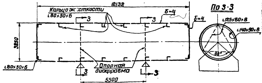
Резервуар 100 м 3 № 704-1-48 (150/2)
