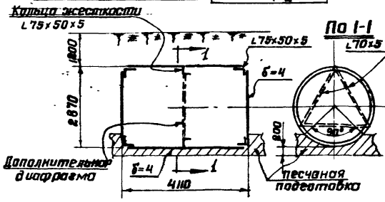
Резервуар 25 м 3 N 704-1-45 (200 п)
