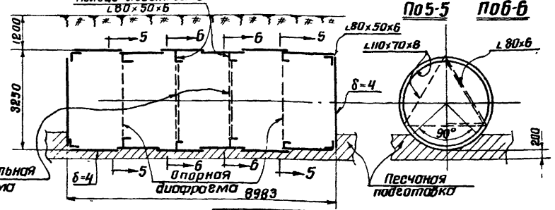
Резервуары 100 м 3 жидк. [704-1-48 ( \frac{150}{1} п)], 704-1-48 ( \frac{150}{1} р п)
