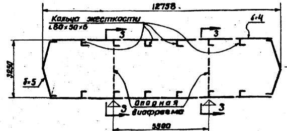
Резервуар 100м³ Н 704-1-48(КА 200/20)
