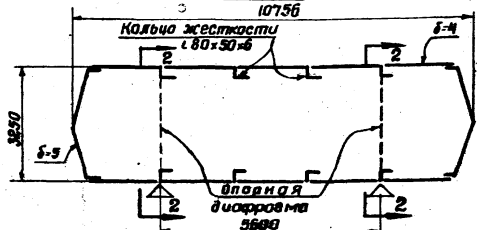
Резервуар 100м³ Н 704-1-48(КА 200/20)
