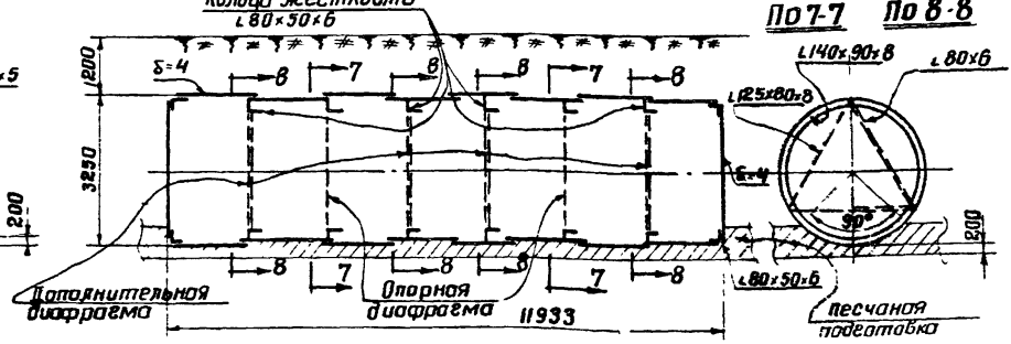
Резервуары 100 м 3 жидк. [704-1-48 ( \frac{150}{1} п)], 704-1-48 ( \frac{150}{1} р п)
