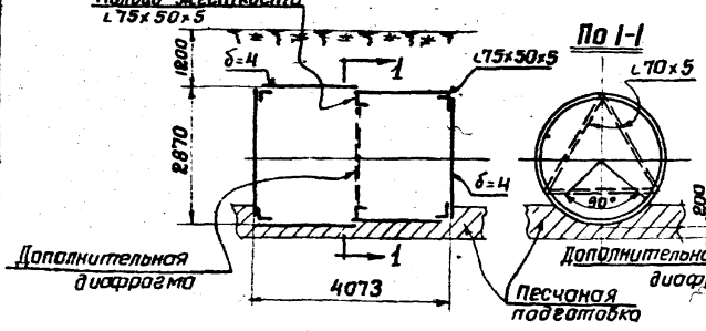
Резервуары 25 3 м 3 704-1-45(200 п) 704-1-45(200 р п) Кольцо жесткости L 75 \times 50 \times 5
