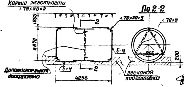
Резервуары 25 м 3 жидк. [704-1-45 ( \frac{140}{1} п)], 704-1-45 ( \frac{140}{1} р п)
