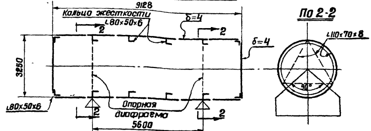
Резервуар 100 м 3 № 704-1-48 (150/2)
