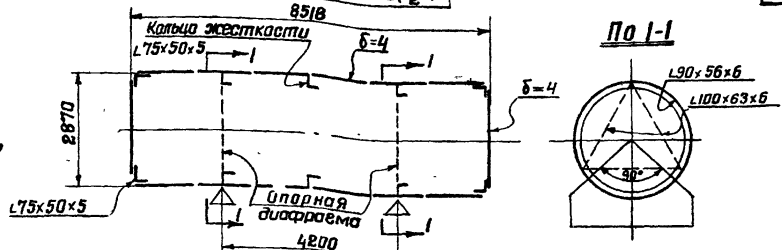
Резервуар 75 м 3 № 704-1-47 (140/2)
