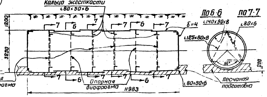
Резервуары 100 3 м 3 704-1-48(200 п) 704-1-48(200 р п) Кольцо жесткости L 80 \times 50 \times 6
