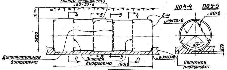
Резервуары 100 3 м 3 704-1-48(200 п) 704-1-48(200 р п) Кольцо жесткости L 80 \times 50 \times 6
