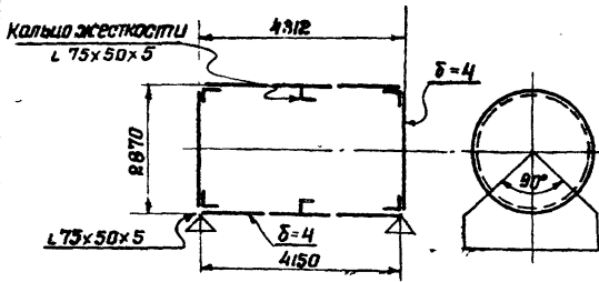
Резервуары
