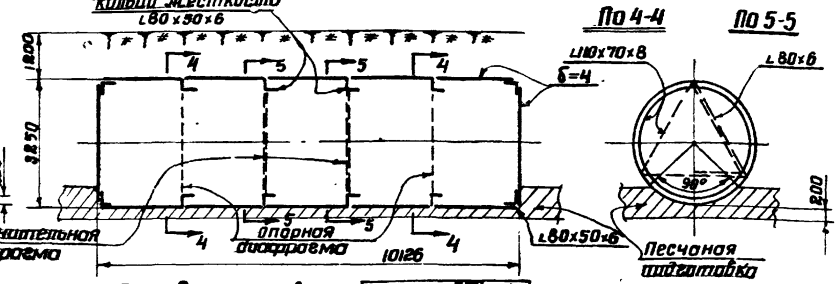
Резервуар 100 м 3 N 704-1-48 (200 п)
