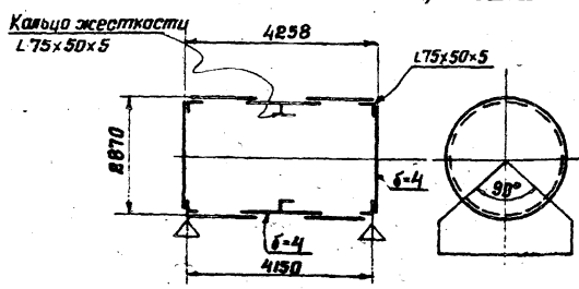
Резервуары 25 м 3 ММ [704-1-45 (140) ], 704-1-45 (150P)
