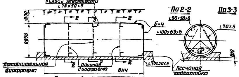
Резервуар 75 м 3 N 704-1-47 (200 п)
