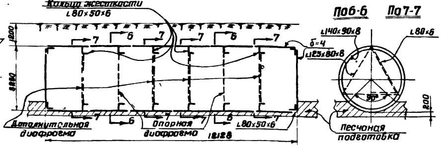
Резервуар 100 м 3 N 704-1-48 (200 п)
