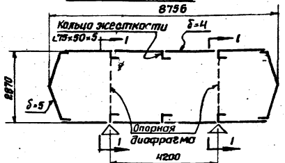
Резервуар 75м³ Н 704-1-47(КА 200/20)
