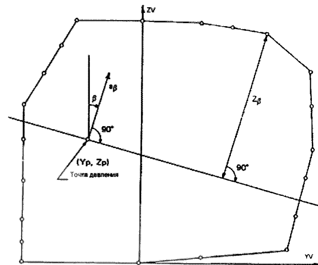
Рис. 3.2.2 Определение внутреннего гидростатического напора
