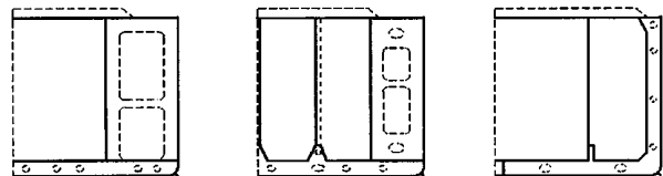
Рис. 2.2.8 Типовые сечения мидель-шпангоута химовоза
