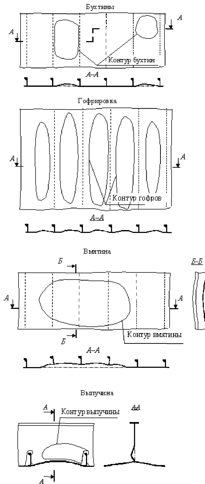
Рис. 1.2.1-1 Виды остаточных деформаций
