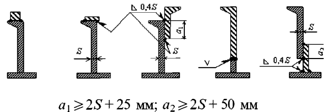
Рис. 5.2.4.1-1 Подкрепления балок набора:
