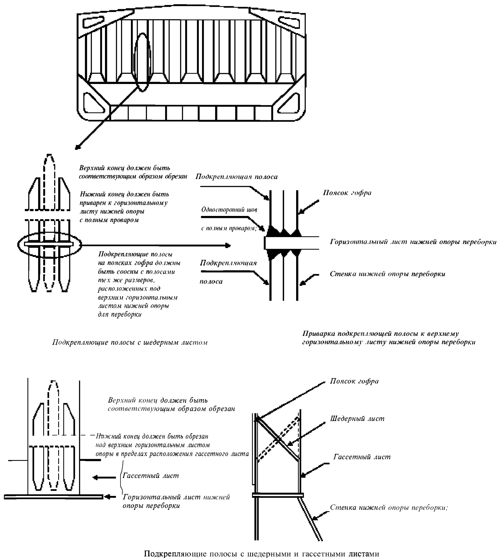
Рис. 1 Общая схема подкрепления переборки.
