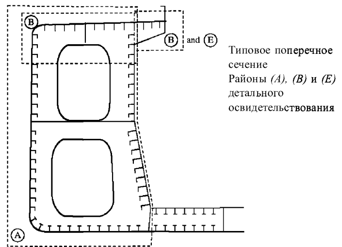
Типовое поперечное сечение Районы (A), (B) и (E) детального освидетельствования
