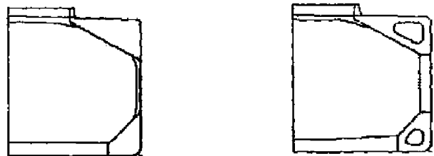
Рис. 2.2.7.3 Типовые сечения мидель-шпангоута нефтерудонавалочного судна
