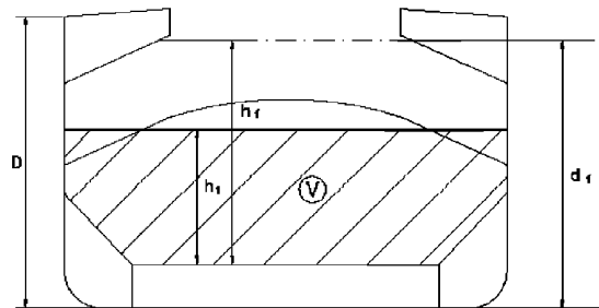
Рис. 5.10.2.2 Схема загруженного трюма ( V — объем груза, м 3 )
