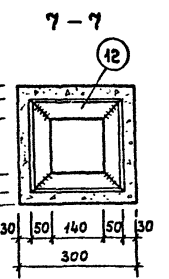
Фундамент Ф-1 (с крышкой)
