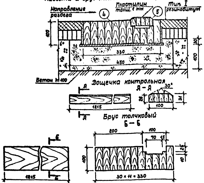
Кассета и брус толчковый в сборе
