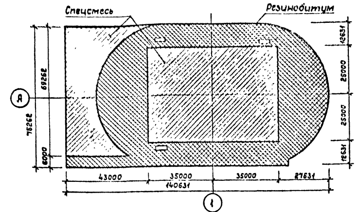
План покрытий
