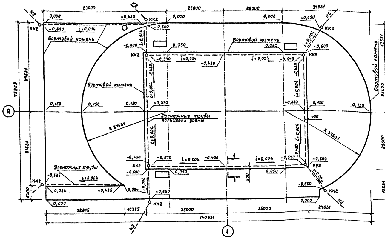
План дренажа
