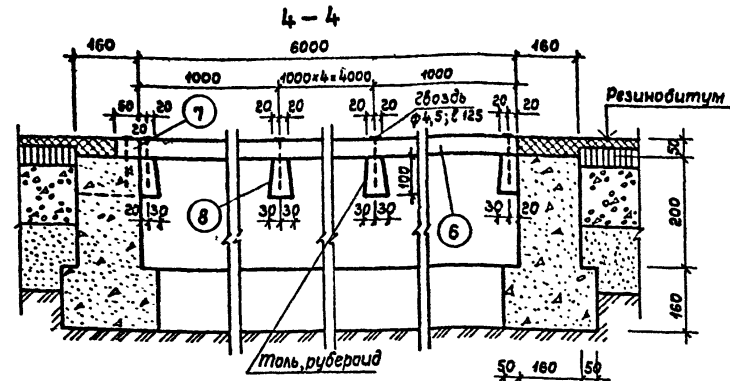
Фундамент Ф-1 (с крышкой)
