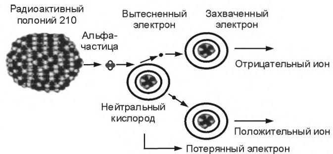
Рисунок 9 — Ионизация альфа-излучением
