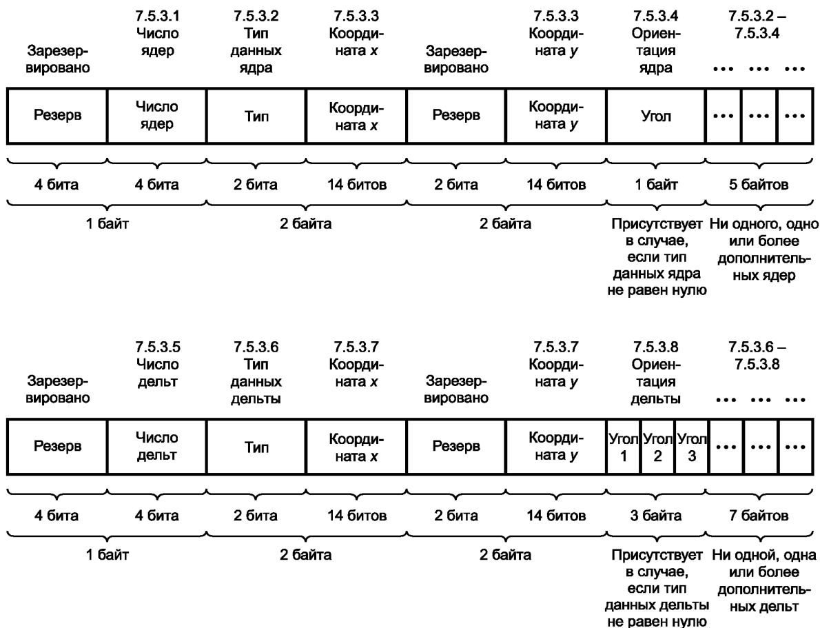
Рисунок 8 — Структура формата данных ядра и дельты
