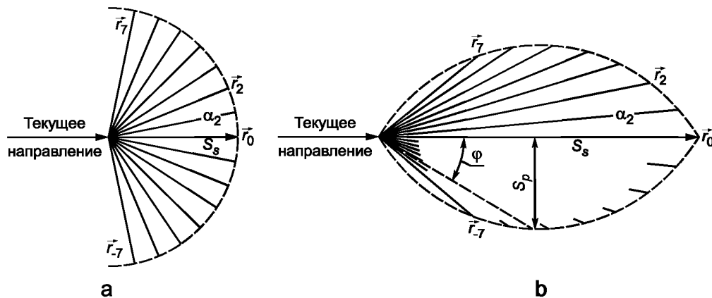
a — при S_p=0 используется постоянная длина шага. В данном случае при угловом разрешении 11,25^\circ ; b — при S_p>0 шаги малых углов изгиба увеличиваются в то время, как уменьшаются шаги больших углов. В данном случае 15 направлений закодировано при высоком угловом разрешении 5,625^\circ .
