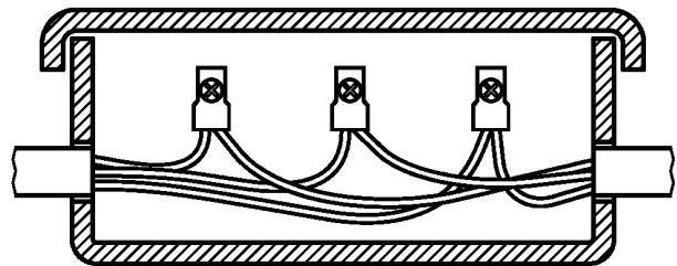
Рисунок АА.1 — Четыре примера соединительных коробок/корпусов
