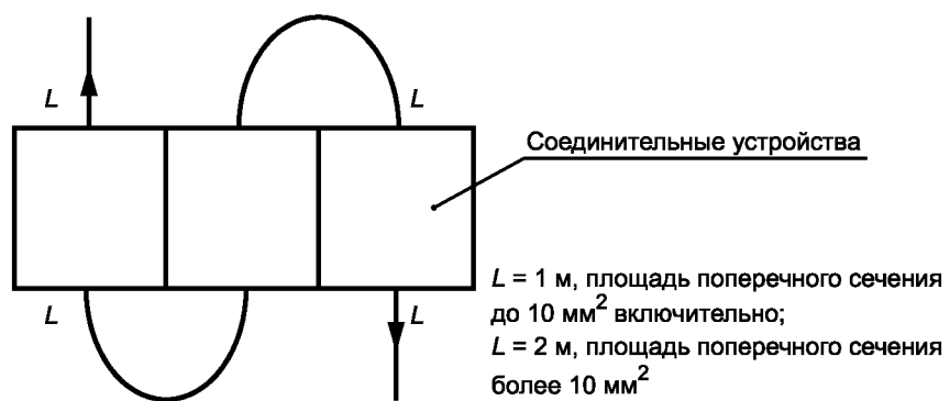
Рисунок 102 — Зажим на несколько направлений
