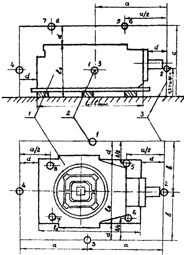
Рис.1.1. Расположение измерительных точек 1 - ротор, 2 - измерительные точки, 3 - измерительная поверхность.
