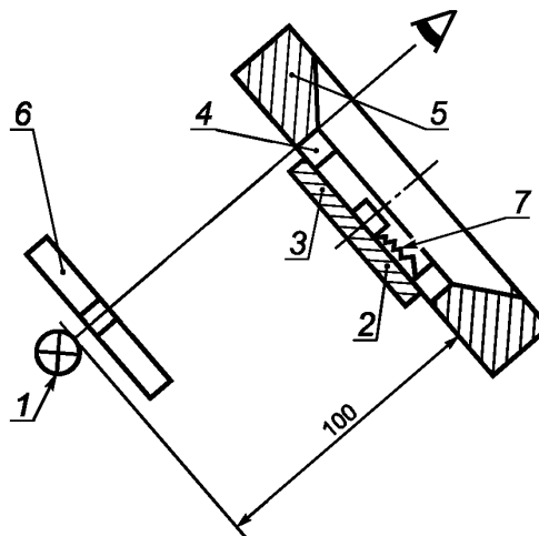
1 — источник света; 2 — непрозрачный экран; 3 — образец просвета; 4 — контролируемое кольцо; 5 — гладкий кольцевой калибр; 6 — фильтр; 7 — имитатор расширителя (расширитель применяют только при контроле колец, работающих с расширителем)
