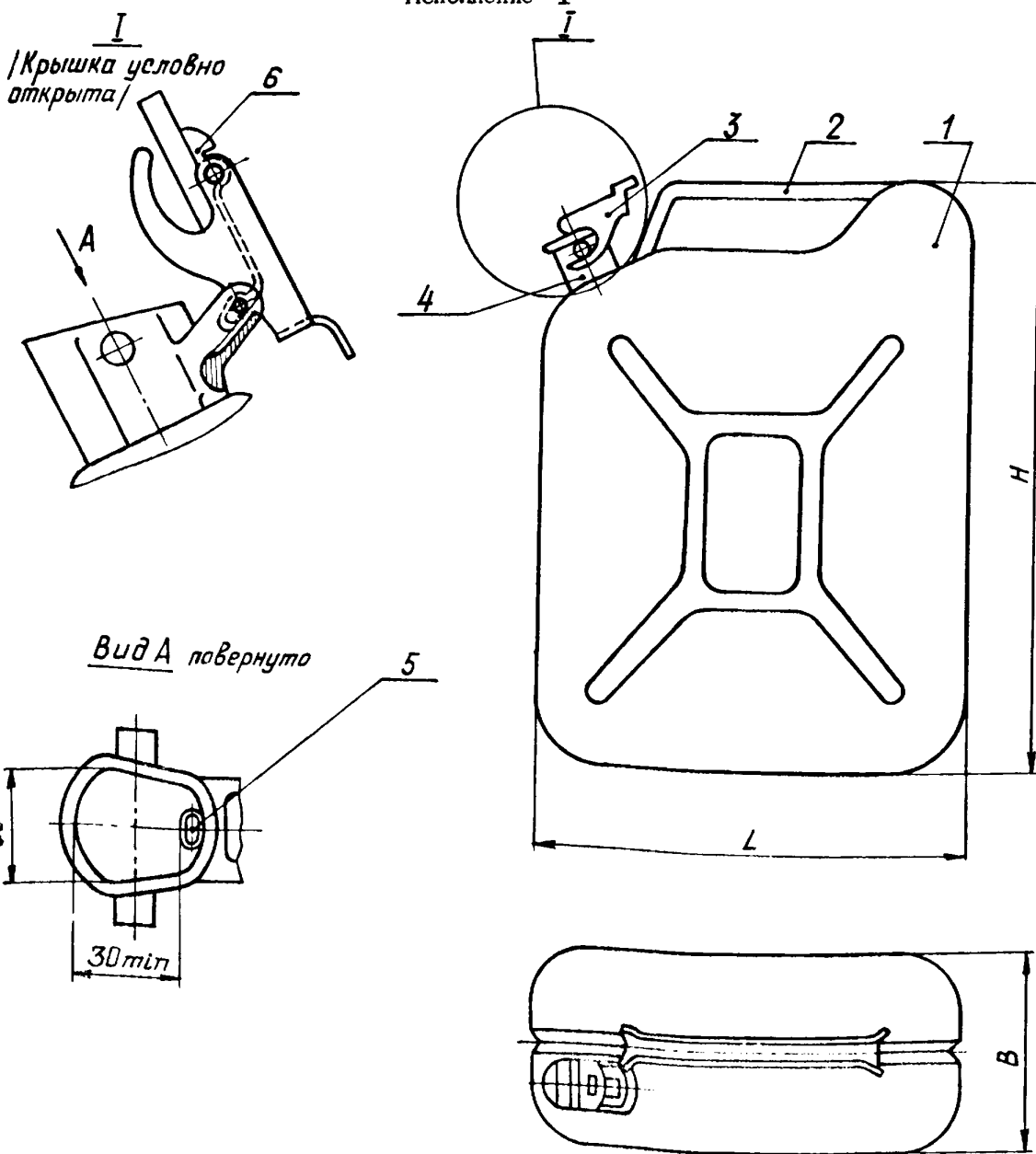
1 - корпус; 2 - ручка; 3 - крышка горловины с рычагом; 4 - горловина; 5 - трубка воздушная; 6 - планка
