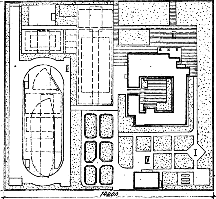
Участок школы на 30 классов (176 уч.)
