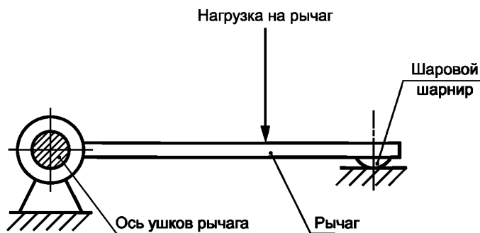
Рисунок 2 — Схема испытаний рычагов на прочность
