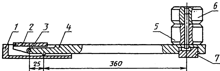
1 — подставка; 2 — коромысло; 3 — ось; 4 — рычаг; 5, 6 — грузы; 7 — амортизатор
