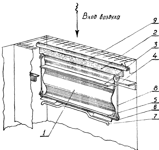
Рис 1. Гибкая подвеска
