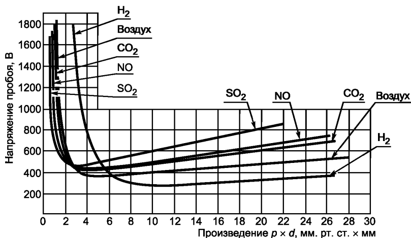
Рисунок 1 — Кривая Пашена
