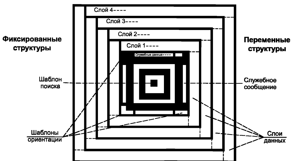
Рисунок 2 — Структура компактного символа Aztec Code
