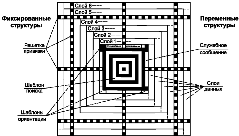
Рисунок 3 — Структура полноразмерного символа Aztec Code
