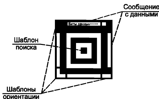
Рисунок А.2 — Структура символа Aztec Rune
