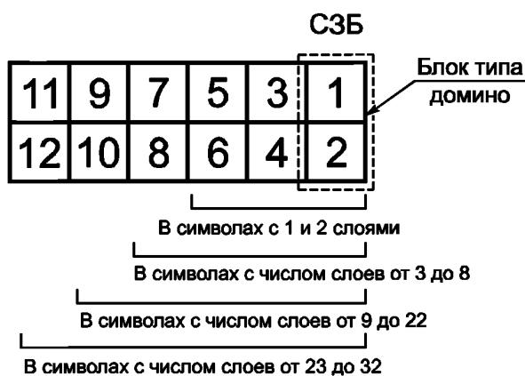
Рисунок 4 — Типовая структура знака в символе 2)
