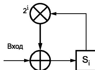
Рисунок В.2 — Схема генерирования значения синдромов
