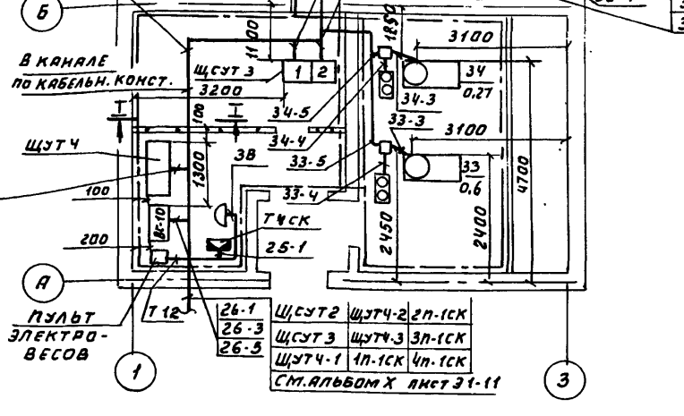
ПЛАН НА ОТМ. 4.200 М 1:100
