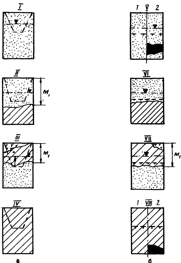
Рис. 3. Типы геологических разрезов, обводняемых при строительстве и эксплуатации трубопроводов:
