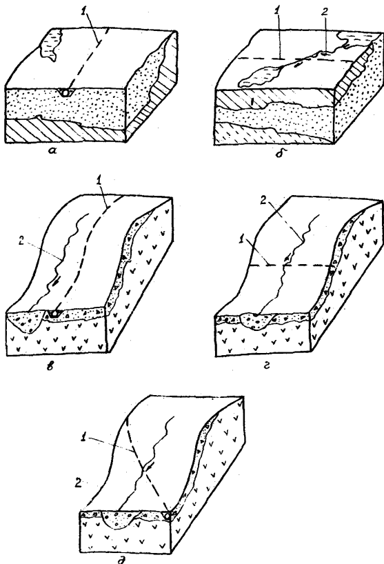
Рис.5. Виды прокладки трубопровода по отношению к рельефу: а - равнинный бесстоковый (рб); б-равнинный поперечностоковый (рс); в-склоновый продольностоковый (сп); г-склоновый поперечностоковый (сч); д-склоновый наклонностоковый (сн); 1-трубопровод; 2 - река, ручей
