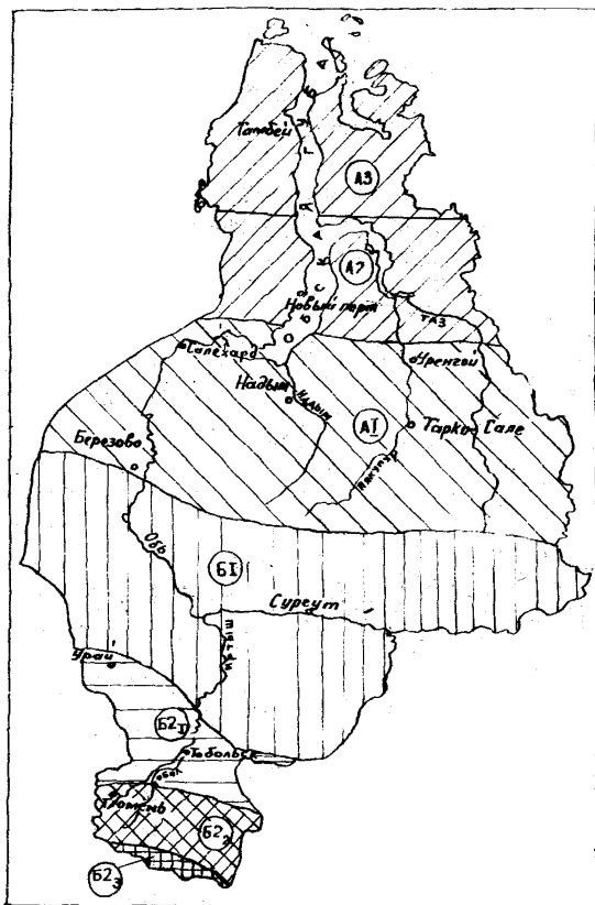
Рис. 5. Мерзотно-гидролого-климатические зоны Тюменской области (за основу взята карта гидролого-климатических зон Тюменской обл. В.С.Мезенцева и И.В.Карнаевича (1971 г.):
