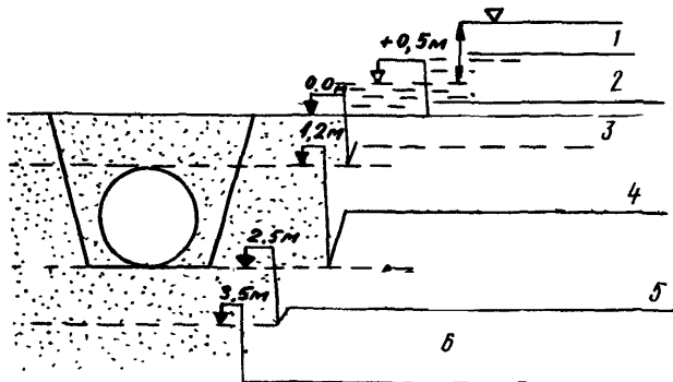
Рис.4. Типы участков по степени обводнения :
