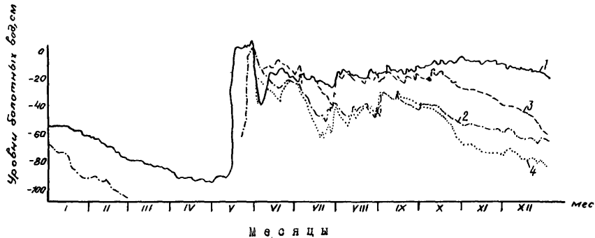
Рис.7. Графики колебаний уровня болотных вод за многоводный 1971 г. (1,3) и маловодный 1969г. (4,2) в пределах зоны А1 (болотный пост Нумто) [II] для различных микроландшафтов: 1,2 - сфагновоосоково-шейхцериевого; 3,4 - сфагново-кустарничково-лишайникового
