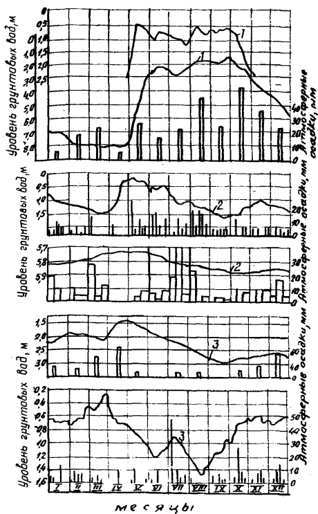
Рис.1. Графики колебаний уровня грунтовых вод в провинциях с различными типами режима [1]:
