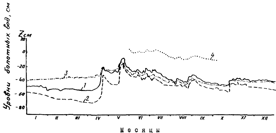
Рис. 8. Графики колебаний уровня болотных вод в пределах зоны Б1 (Самотлорский болотный массив, 1970 г.) [II] для различных микроландшафтов: 1 - сфагново-кустарничково-соснового; 2 - сфагново-кустарничкового, облесенного сосной; 3 - грядово-мочажинного (гряда); 4 - грядово-мочажинного (мочажина)
