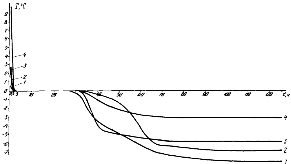
Рис. II. Изменение температур на различных горизонтах скважины № 2 ( l_{\text{СКВ}} ) пос. Малая Хета: 1 - l_{\text{СКВ}} = 5,0 м; 2 - l_{\text{СКВ}} = 4,5 м; 3 - l_{\text{СКВ}} = 3,5 м; 4 - l_{\text{СКВ}} = 2,0 м
