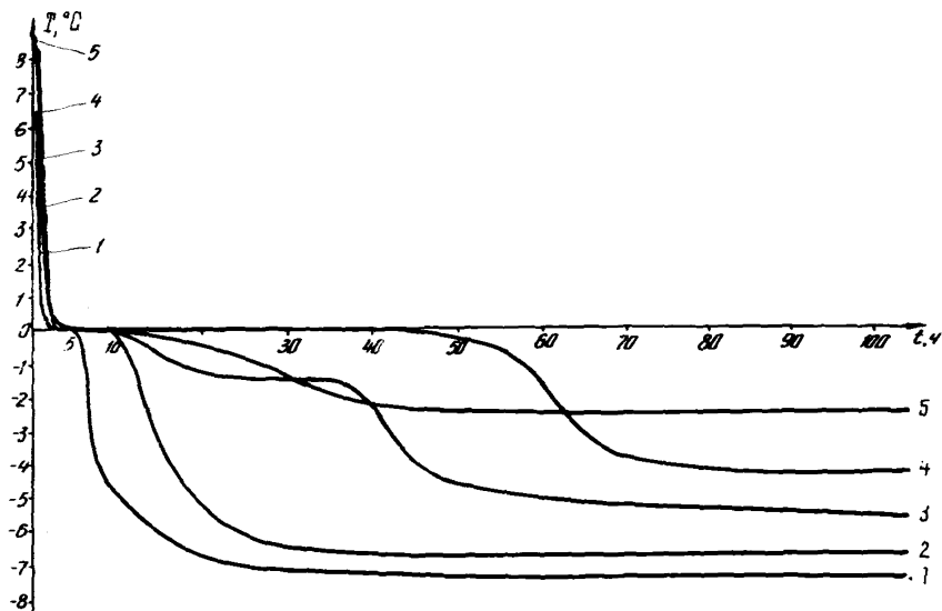
Рис. 10. Изменение температур на различных горизонтах скважины № I ( l_{\text{СКВ}} ) пос. Малая Хета: 1 - l_{\text{СКВ}} = 3,3 м; 2 - l_{\text{СКВ}} = 2,5 м; 3 - l_{\text{СКВ}} = 1,8 м; 4 - l_{\text{СКВ}} = 1,3 м; 5 - l_{\text{СКВ}} = 0,8 м
