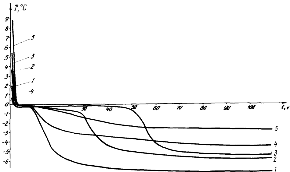
Рис.12. Изменение температур на различных горизонтах скважины № 3 ( l_{\text{СКВ}} ) пос.Малая Хета: 1 - l_{\text{СКВ}} = 3,0 м; 2 - l_{\text{СКВ}} = 2,5 м; 3 - l_{\text{СКВ}} = 2,0 м; 4 - l_{\text{СКВ}} = 1,0 м; 5 - l_{\text{СКВ}} = 0,5 м
