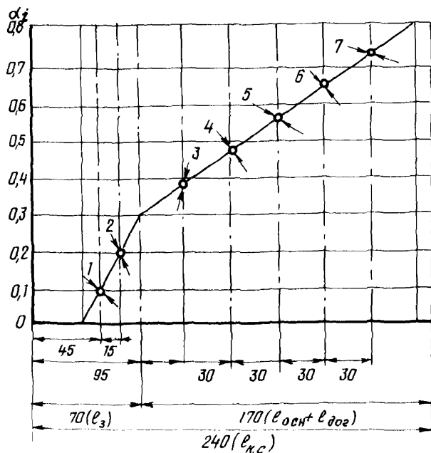
Рис.7. Схема расчета отверстий для подачи воздуха в камеру сгорания термобура ТВВД-107м:
