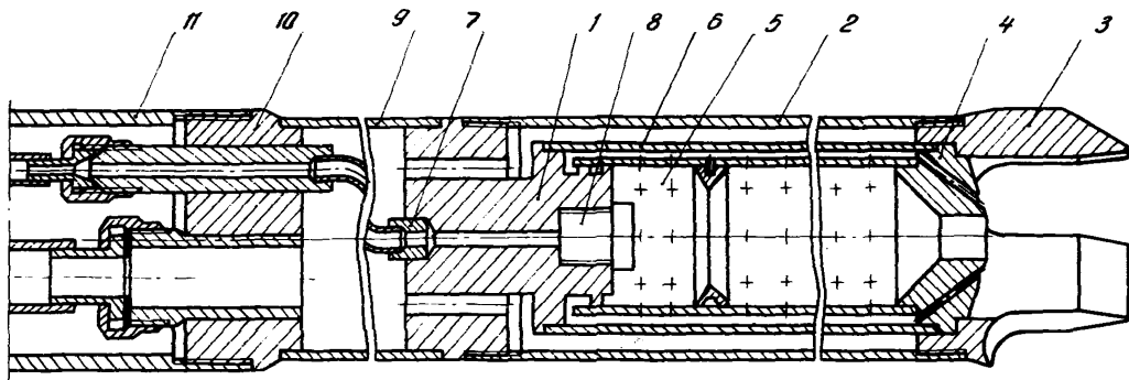
Рис.3. Термобур ТВЦ-107М:
