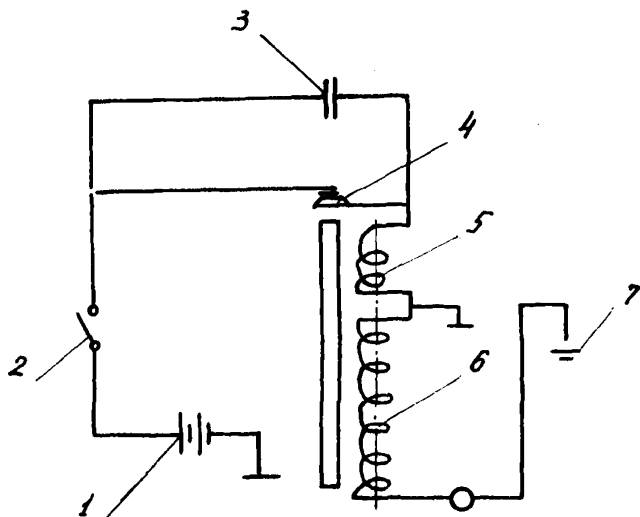
Рис.5. Схема электрозажигачего устройства: 1-источник питания; 2-кнопочный выключатель; 3-конденсатор; 4-контакт; 5,6-преобразователи напряжения; 7-запальная свеча
