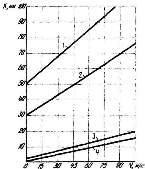
Рис. 9. Влияние начальной скорости ввода струи воздуха и топливной смеси на положение зоны дожигания в факеле при разном количестве струй \{ n \} и угла их ввода \{ \beta \} :
