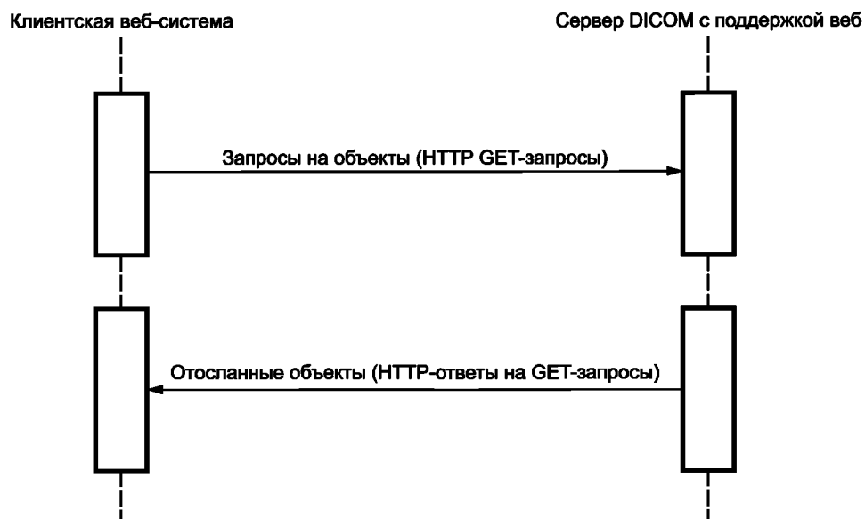
Рисунок 1 — Схема взаимодействия
