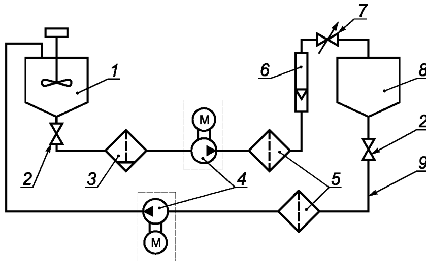
Схема установки для определения полноты отделения воды
