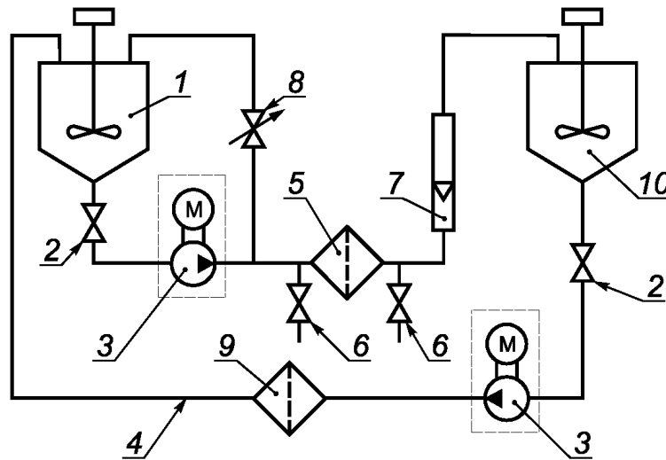
Схема установки для определения полноты отсева фильтром
