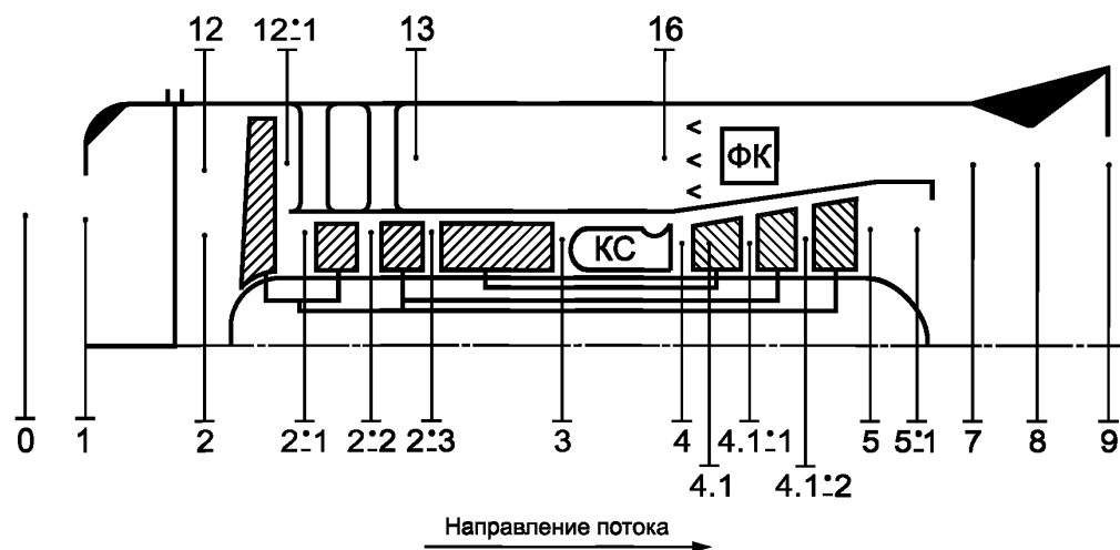
Рисунок 2 — Схема нумерации контрольных сечений для двигателей ТРДДФ со смещением контуров и общим соплом
