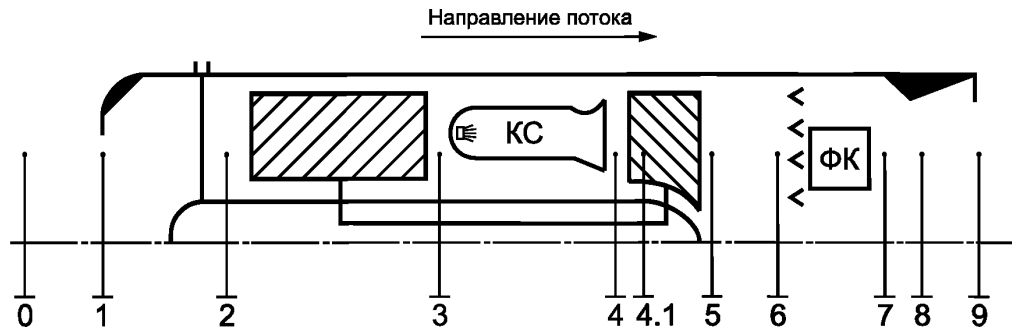
Рисунок 1 — Базовая СНКС для двигателя ТРДФ Нумерация сечений — см. таблица 1
