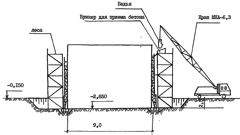
Схема погружения ошусного колодца в связных грунтах
