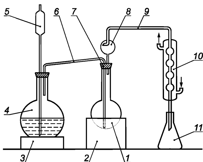
1 — колба Гр—250—14/23 ТС по ГОСТ 25336 с анализируемой пробой; 2 — колбонагреватель электрический мощностью 200—400 Вт; 3 — электрическая плитка по ГОСТ 14919; 4 — колба П—1—2000—29/32 по ГОСТ 25336 с водой (парогенератор); 5 — предохранительная трубка (водяной затвор); 6, 9 — паропроводные трубки внутренним диаметром 6 мм; 7 — пробка; 8 — каплеуловитель КО—60 ХС по ГОСТ 25336; 10 — холодильник ХШ-3/200 ХС по ГОСТ 25336; 11 — приемная колба Кн—1-250-29/32 по ГОСТ 25336
