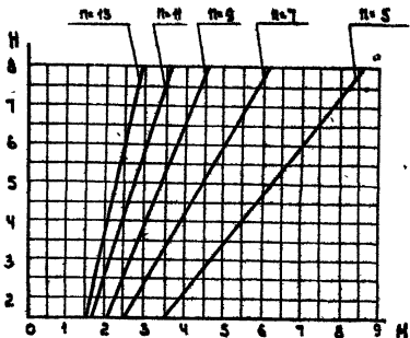
Рис. 3.1. Расчетный момент от поперечного удара.
