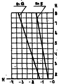
Рис. 3.4. Расчетная продольная растягивающая сила от ледовой нагрузки.
