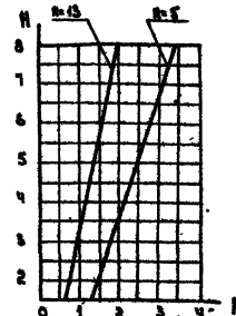
Рис. 3.6. Расчетная продольная сжимающая сила от ледовой нагрузки.
