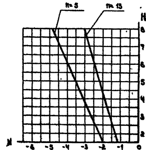
Рис. 3.3. Расчетная продольная сжимающая сила от поперечного удара.
