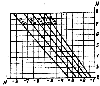
Рис. 4.5. Расчетная продольная растягивающая сила от поперечного удара
