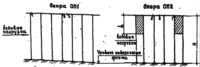
Рис. 8. Расположение расчетных сечений в насадке.
