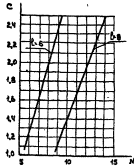
Рис.1.2. Расчетная продольная минимальная сила от постоянной нагрузки
