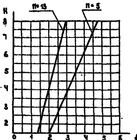
Рис. 3.5. Расчетная продольная сжимающая сила от поперечного удара
