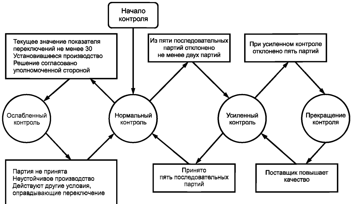
Рисунок 1 — Схема правил переключения (см. 10.3)
