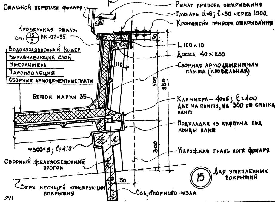
ТА 1956 Деталь 15. Нижний борт П-образного фонаря из сборных армированных кровельных плит длиной 3 м (в покрытиях по сборным железобетонным прогонам). ПК-02-21 Лист II
