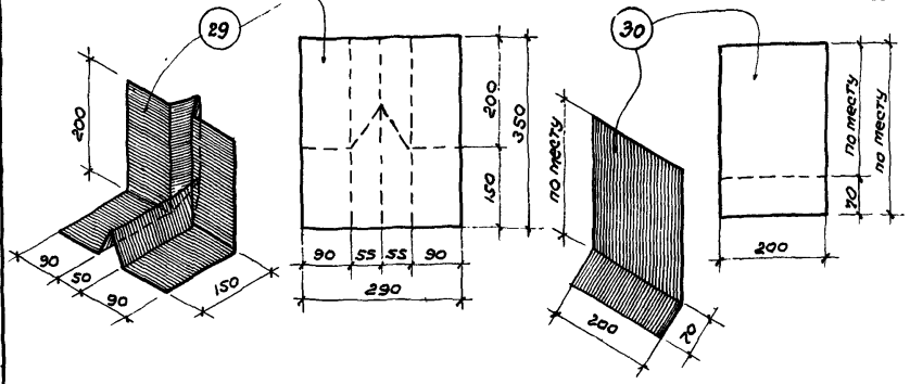
Аксонотрия и раскрой элементов 29 и 30
