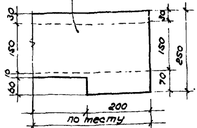
Аксонометрия и раскрой элемента 32
