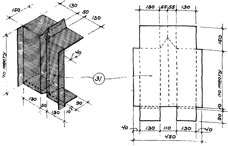
Аксонометрия и раскрой элемента 31
