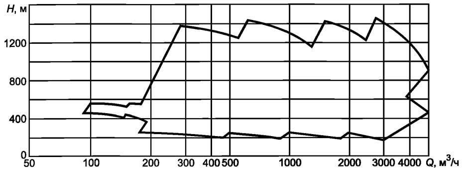
Рисунок Б.2 — Совмещенные поля Q - H магистральных нефтяных полнапорных насосов
