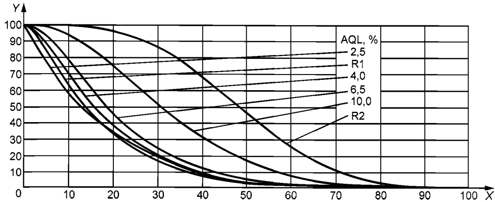
X — качество процесса (в виде процента несоответствующих единиц продукции); Y — средний процент принятых партий
