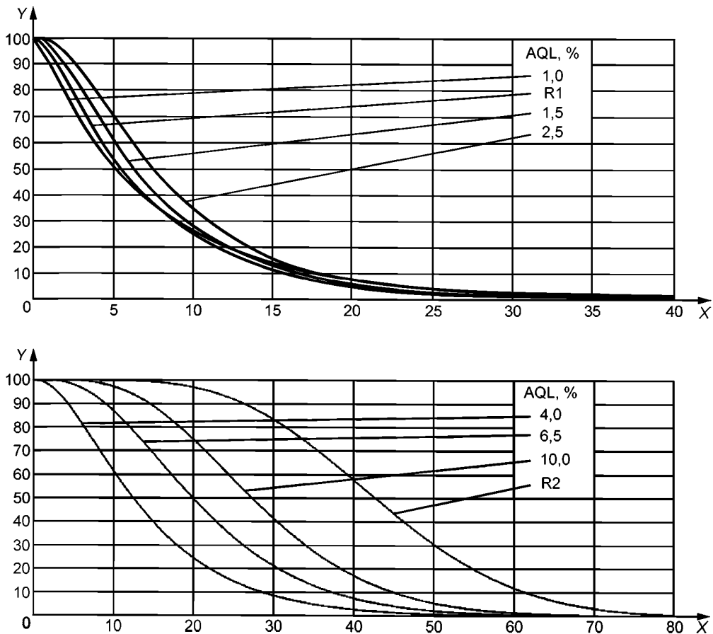
X — качество процесса (в виде процента несоответствующих единиц продукции); Y — средний процент принятых партий
