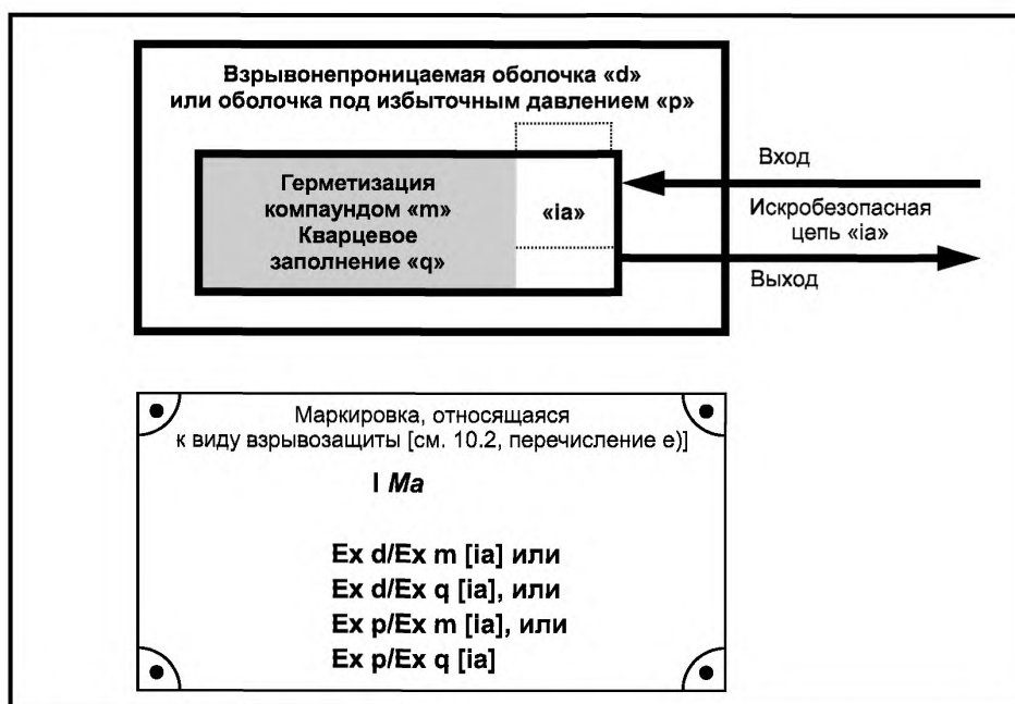
Рисунок 3 — Оборудование уровня взрывозащиты Ma (герметизация компаундом «т» и кварцевое заполнение «q» внутри взрывонепроницаемой оболочки «d» или оболочки под избыточным давлением «р»)
