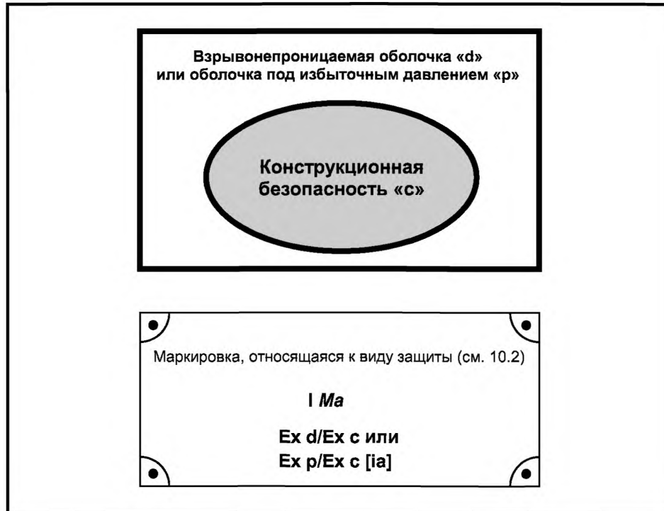
Рисунок 5 — Оборудование уровня взрывозащиты Ma (конструкционная безопасность «с» внутри взрывонепроницаемой оболочки «d» или оболочки под избыточным давлением «p»)
