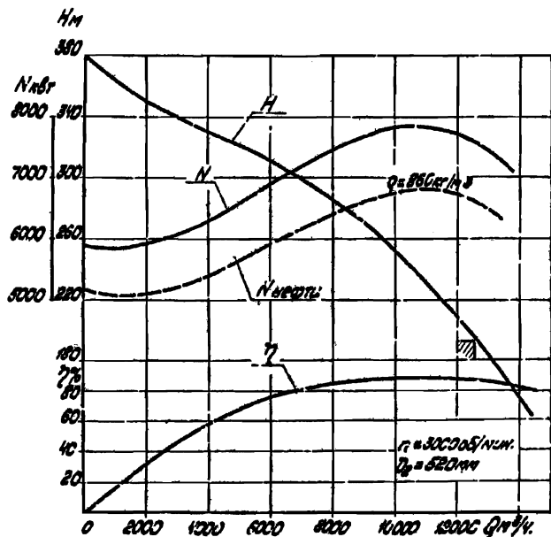
Рис.14. Характеристика нефтяного центробежного насоса БН 10000-210 с ротором 12500 \text{м}^3/\text{ч}
