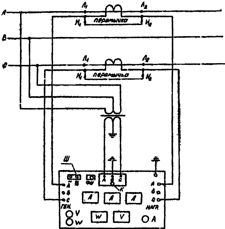
Рис. 1. Схема включения комплекта К-51 при напряжениях 5 и 10 кВ
