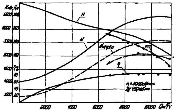
Рис. 13. Характеристика насоса NI 10000-210 по результатам заводских испытаний: \circ - точки, полученные при промышленных испытаниях
