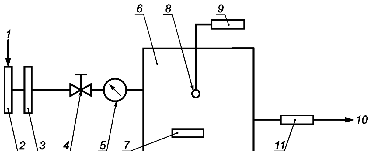
Схема установки с испытательной камерой
