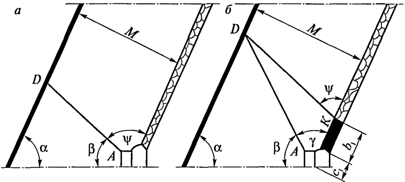
Рис. 1. Схема к определению направления скважины, буримой из откаточного штрека на вышележащий сближенный пласт в плоскости, нормальной к простиранию пласта: a — при отсутствии целика (бутовой полосы) над штреком; б — при наличии целика (бутовой полосы) над штреком
