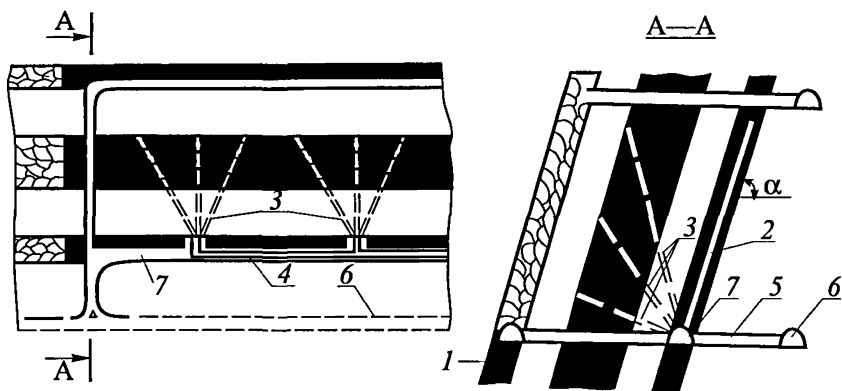
Рис. 15. Схема дегазации свиты крутых пластов скважинами, пробуренными веером вкрест одного пласта и в плоскости другого: 1 — отработываемый пласт; 2 — пластовые дегазационные скважины; 3 — дегазационные скважины, пробуренные вкрест пласта; 4 — газопровод; 5 — квершлаг; 6 — полевой штрек; 7 — откаточный штрек
