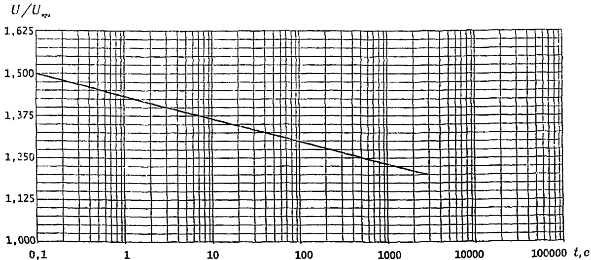
Рис.7. Зависимость "допустимое напряжение-время" для случая предварительного нагружения импульсом 2,25 \text{ кДж/кВ } U_{нрз} для ОПН, выпускаемых ООО "Таврида-Электрик" по ТУ № ИТБА 674361.0005.
