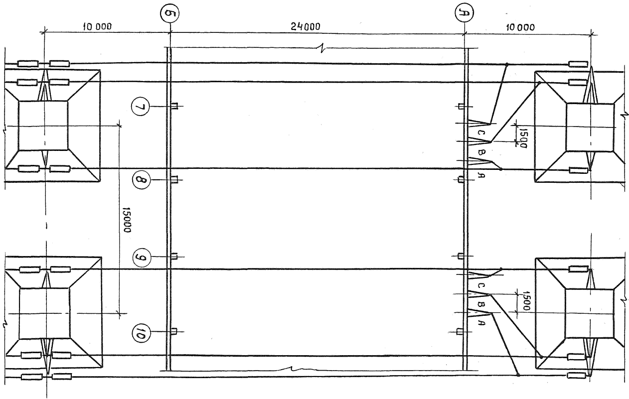
Пример перехода ошиновки над зданием ЗРУ. План (вариант с унифицированными анкерно-угловыми опорами типа УИ10-1+4)
