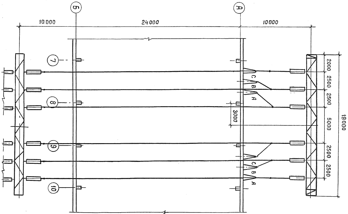
Пример перехода ошиновки 110 кВ над зданием ЗРУ. План (вариант с порталами, выполненными аналогично порталу ПС-500-Л6)
