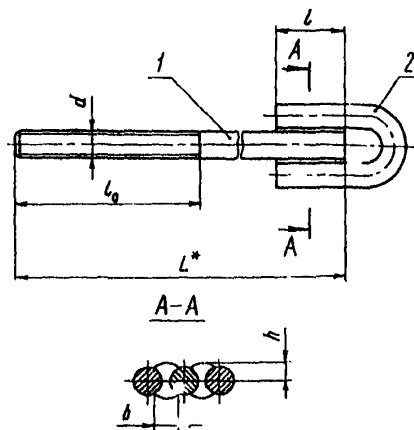
1 — тяга резьбовая; 2 — ушко
