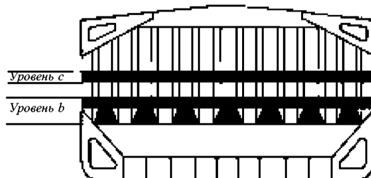
Рис. 2 Уровни b и с для замеров толщин поперечной переборки, имеющей нижнюю опору:
