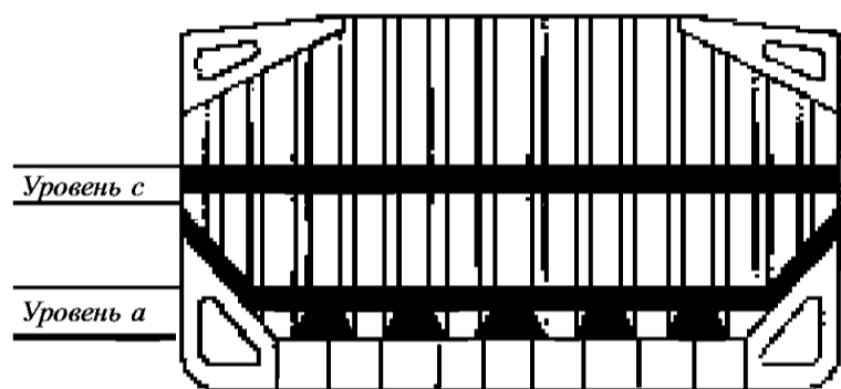
Рис. 1 Уровни а и с для замеров толщин поперечной переборки, не имеющей нижней опоры:
