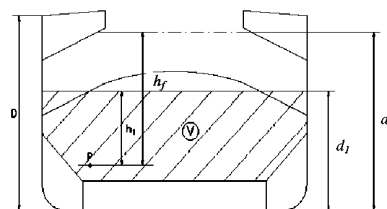
Рис. 5.9.2.2 Схема загруженного трюма ( V — объем груза м 3 ; P — расчетная точка)
