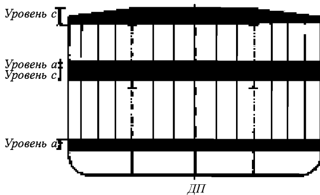
Рис. 7.2.3.2-3 Уровни а и с детальных освидетельствований поперечной переборки твиндечного грузового трюма на судах, предназначенных для перевозки сухих генеральных грузов
