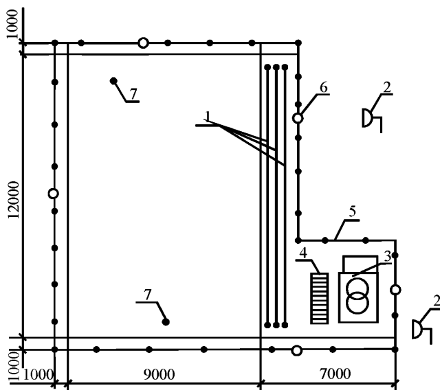
1 – инвентарная трехфазная секция шинопроводов; 2 – прожектор; 3 – трансформаторная подстанция КТП ТО-80/86 с инвентарным распределительным устройством; 4 – диэлектрический коврик; 5 – инвентарное ограждение рабочей зоны; 6 – сигнальная лампочка красного цвета; 7 – температурные датчики
