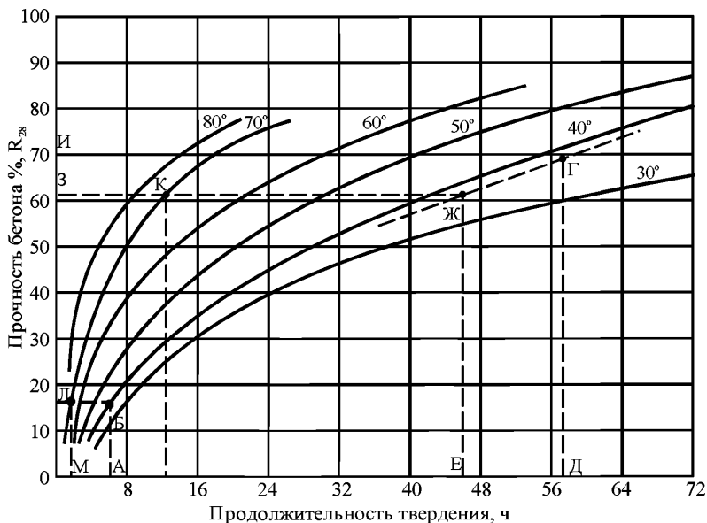
Рисунок 7 – Пример определения прочности бетона по графику
