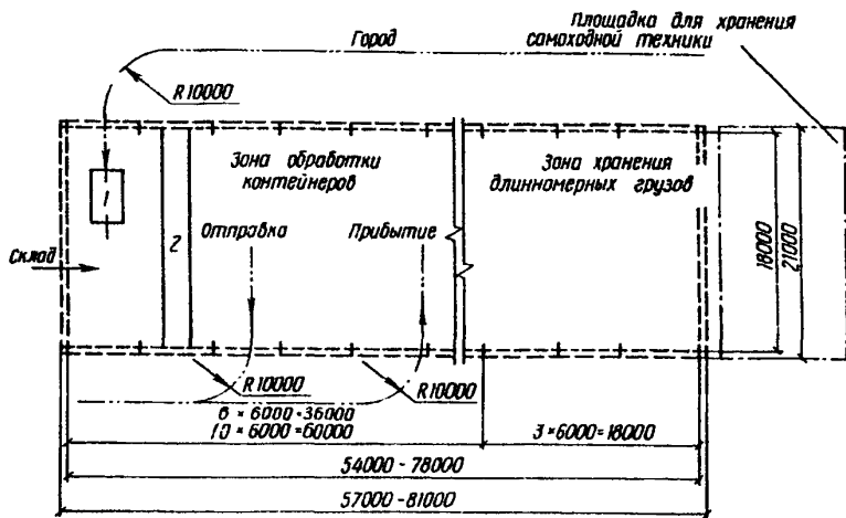
Рис. 16. Схема размещения оборудования на контейнерной площадке с грузооборотом до 120 т/сут. (для аэропортов Крайнего Севера): 1 — весы передвижные автомобильные грузоподъемностью 10 т; 2 — край мостовой грузоподъемностью 20 т
