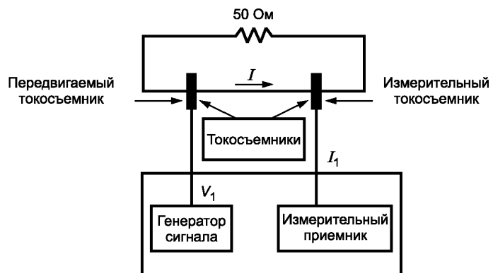
Рисунок А.5 — Схема калибровки
