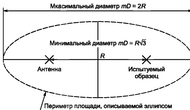
Рисунок 1 — Размеры рабочей зоны измерительной площадки
