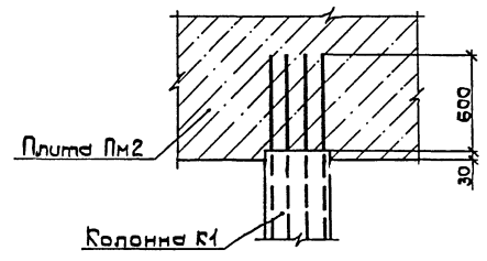
Узел сопряжения колонны K1 с плитой ПМ2
