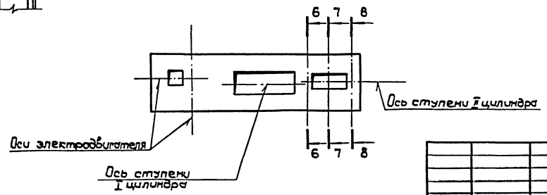
Местоположение разрезов
