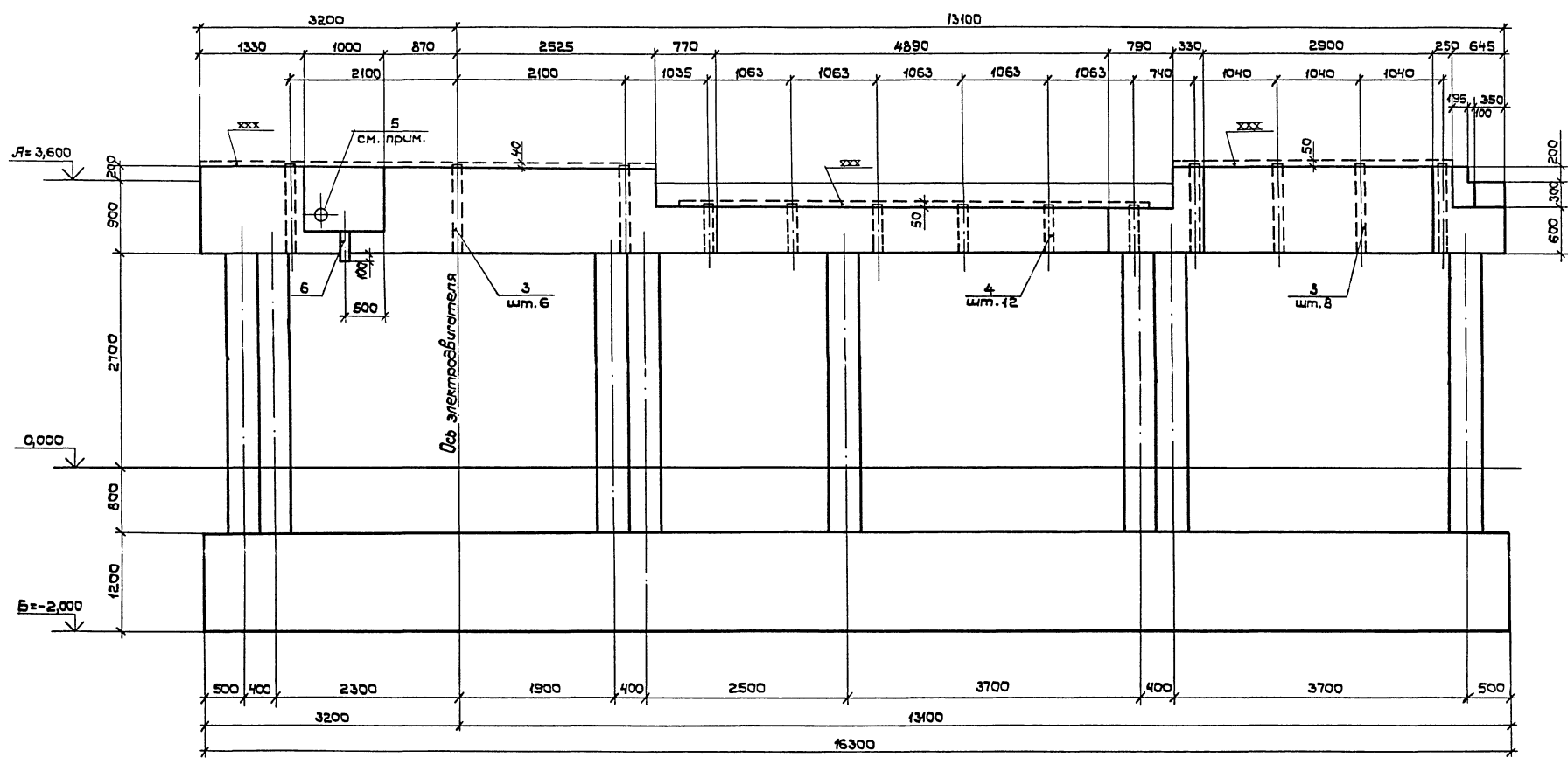
Местоположение разрезов
