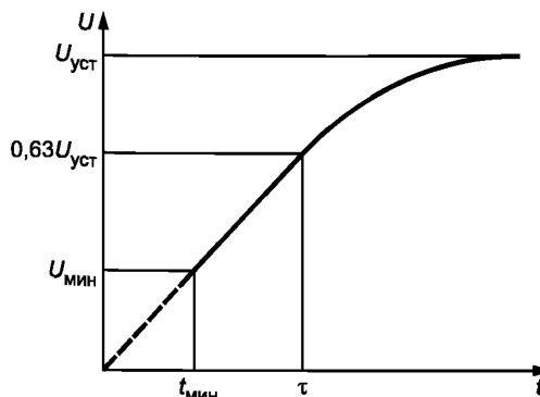
Рисунок 2 — Кривая натекания
